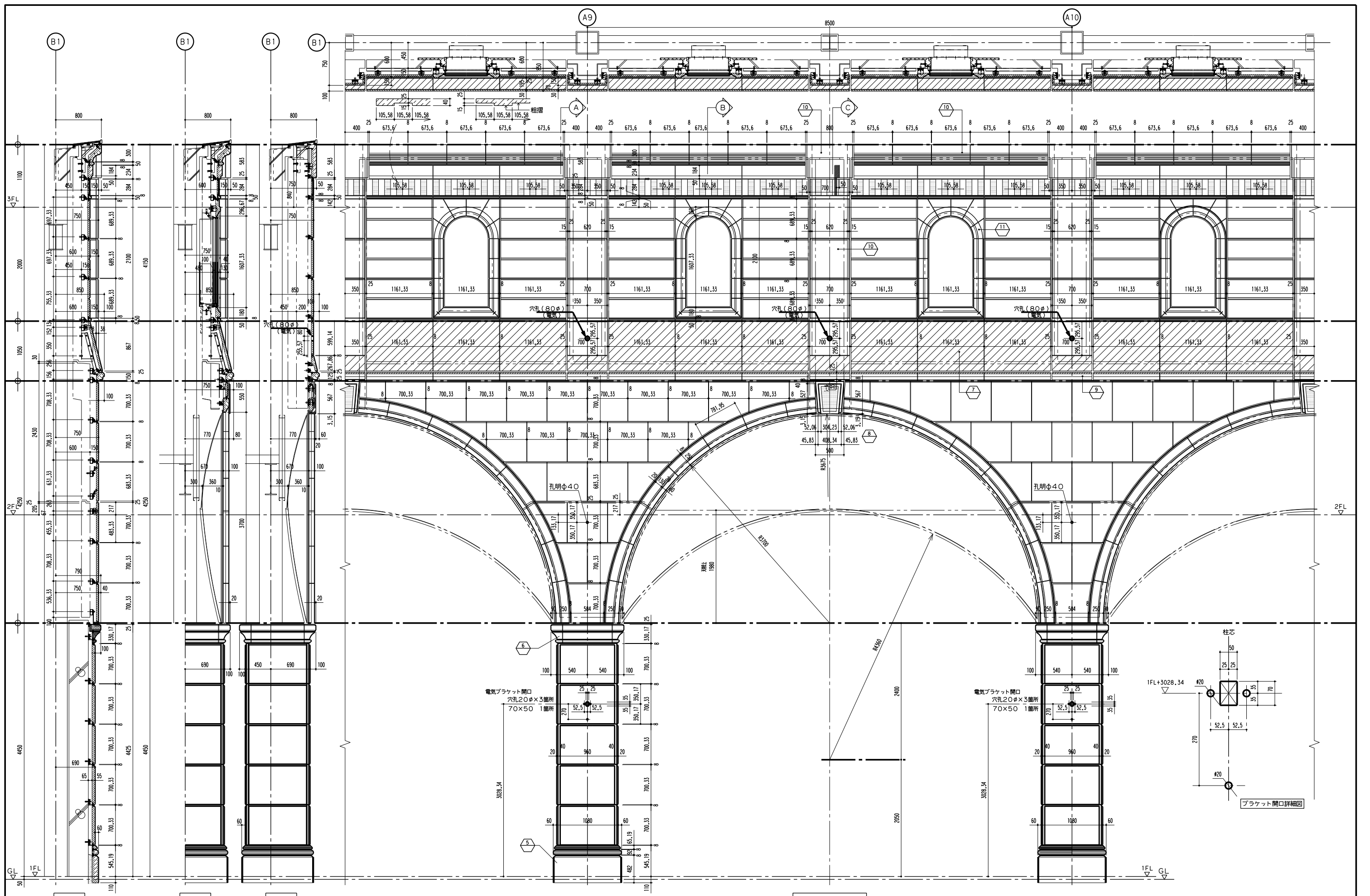
低層南立面図 S=1/30
